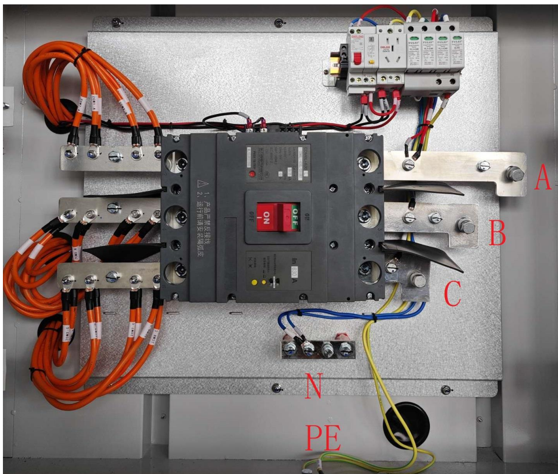
充电机交流进线安装位置图
