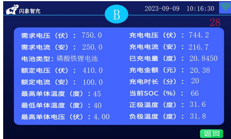
充电过程数据显示图
